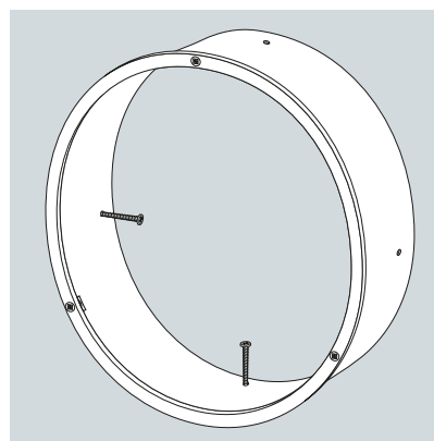
Einbauahmen 01.460.300 für u.P.-Montage in konventionellen Mauerwerkswänden
